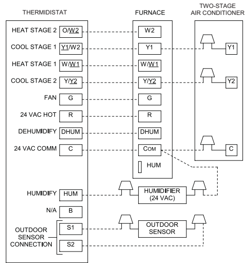
Thermostat modèle TSTATBBPRH01-B avec appareil de chauffage VS et climatiseur 2 étages
