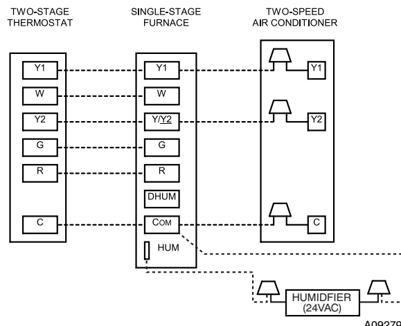
Thermostat 2 étages avec appareil de chauffage 1 étage et climatiseur 2 étages
