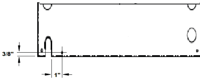
Fig. 2 – Deep Door Furnace / Blower Door Switch Location
