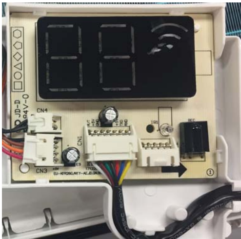
Figure 4 – Raccordez le connecteur JST
