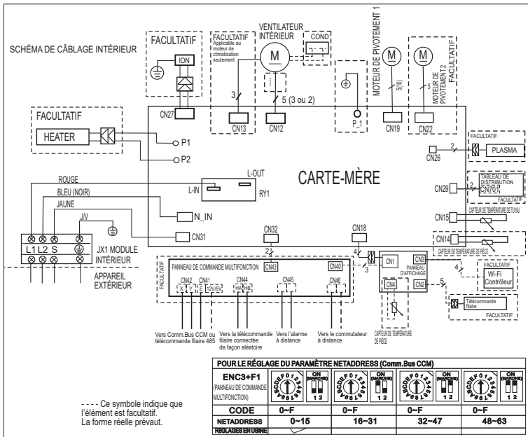
Figure 2 – 230V Montage mural élevé, niveau d'entrée SEULEMENT
