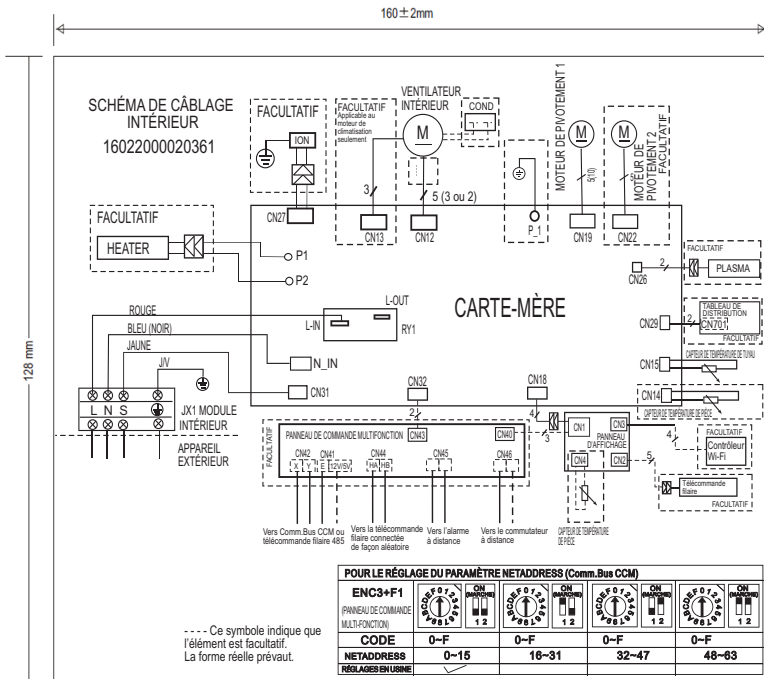
Figure 1 – 115V Montage mural élevé, niveau d'entrée SEULEMENT
