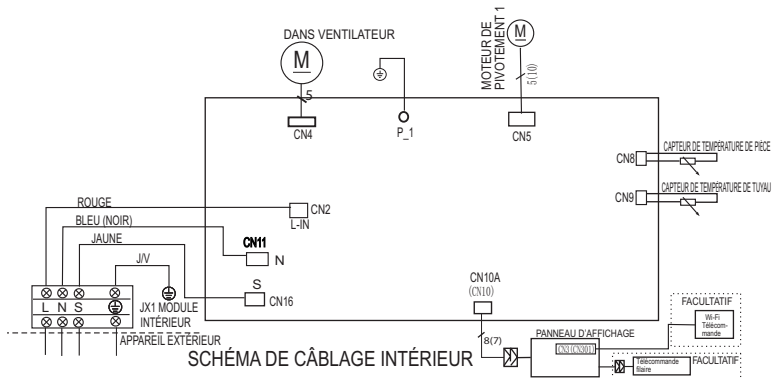
Figure 3 – Montage mural niveau moyen SEULEMENT
