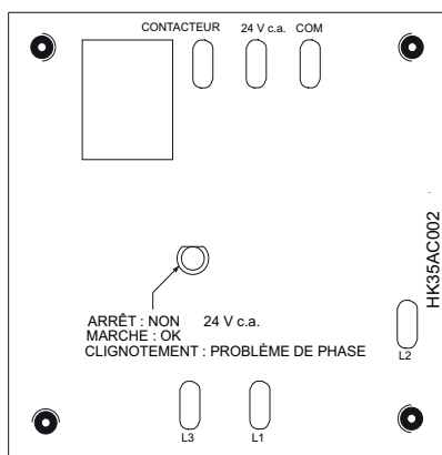
Fig. 7 – Commande de moniteur triphasé (s'applique aux appareils triphasés seulement)
