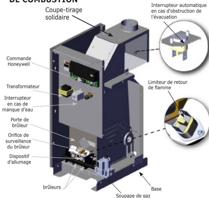
FIGURE 2 – VOIES DE PASSAGE DES RÉSIDUS DE COMBUSTION
